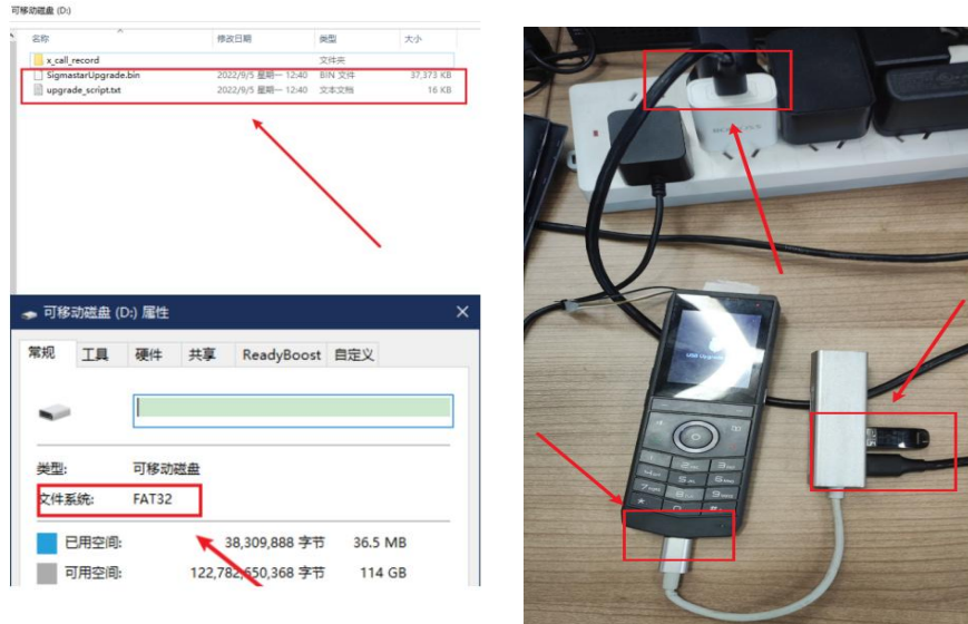
图 151 - U 盘升级所需的准备
