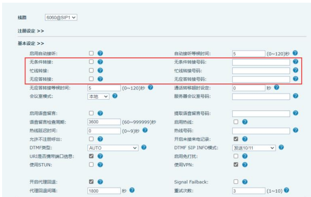
图 44 - 设置呼叫前转
